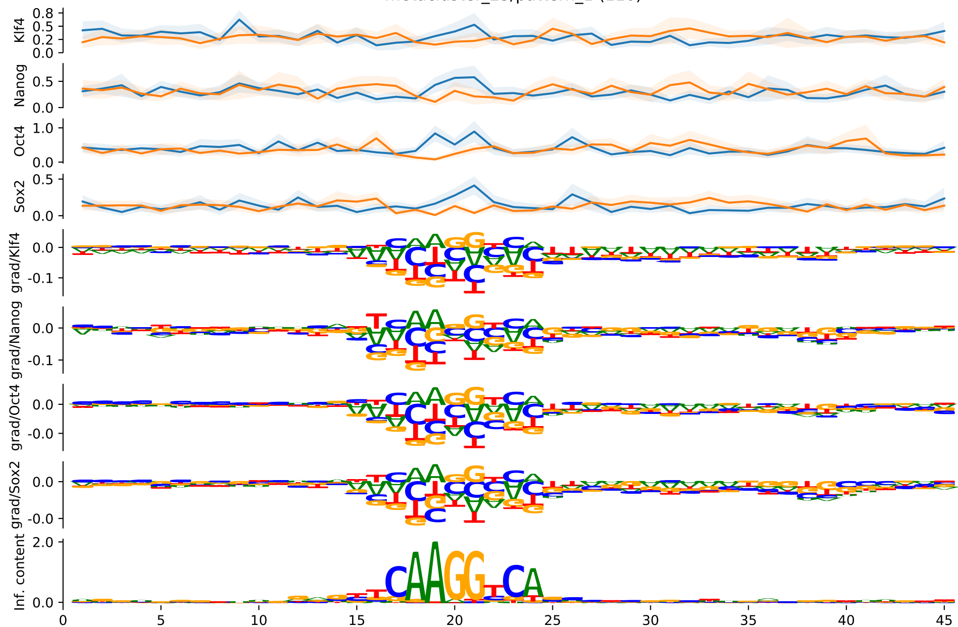
metacluster_23/pattern_1 (110)
