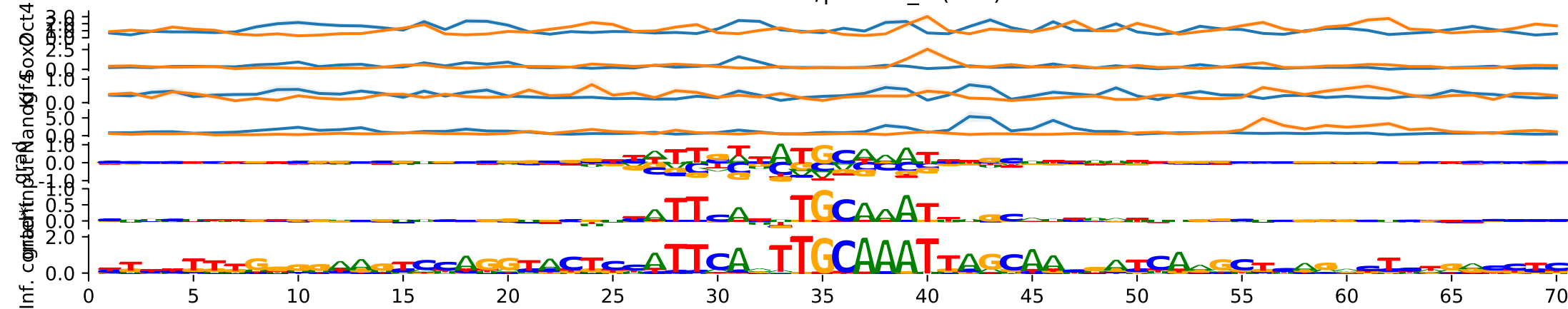
metacluster0/pattern_6 (158)
