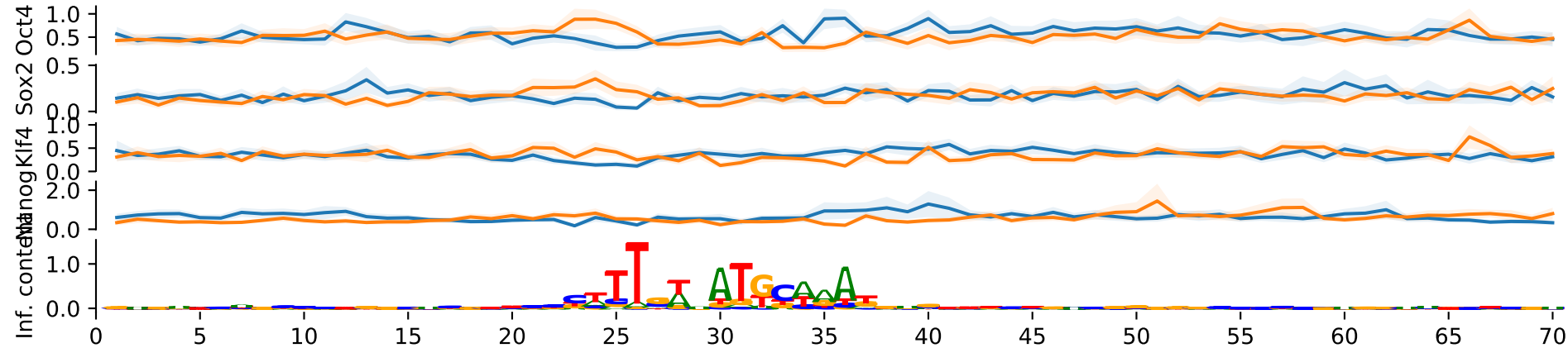
motif 3 (201)
