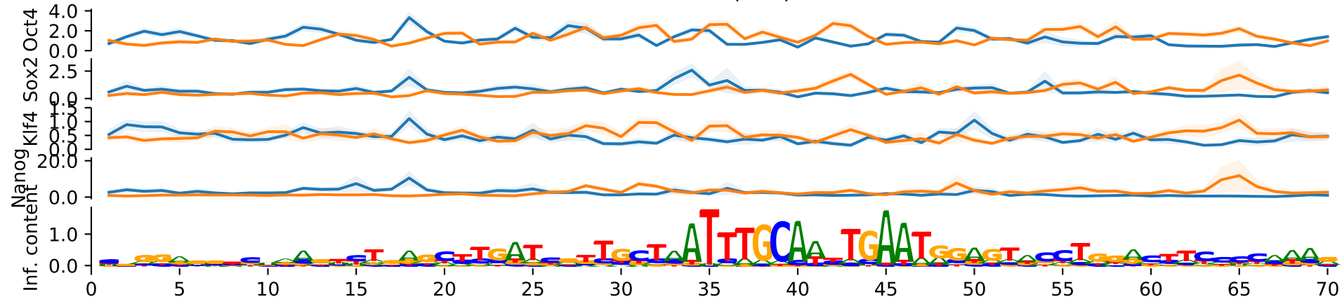
motif 5 (187)
