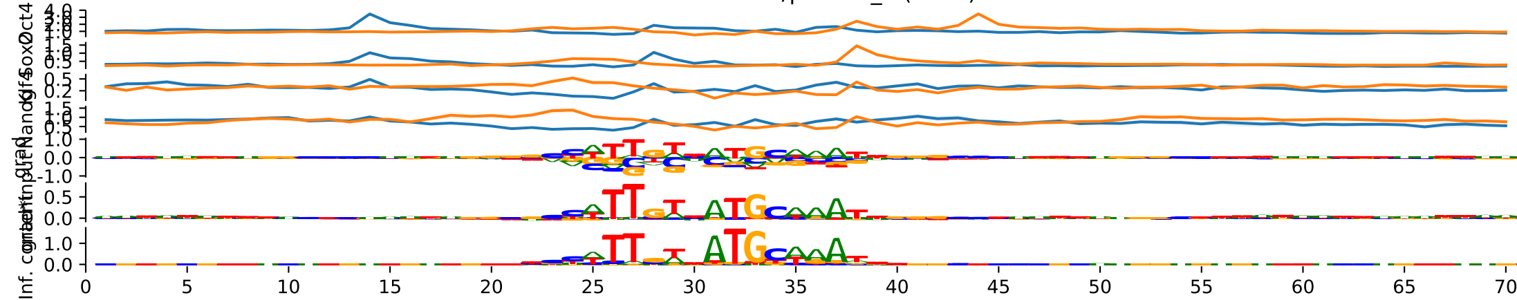
metacluster0/pattern_1 (1903)
