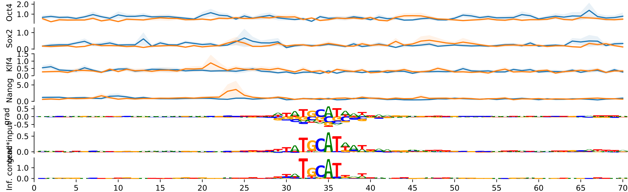
metacluster0/pattern_6 (195)
