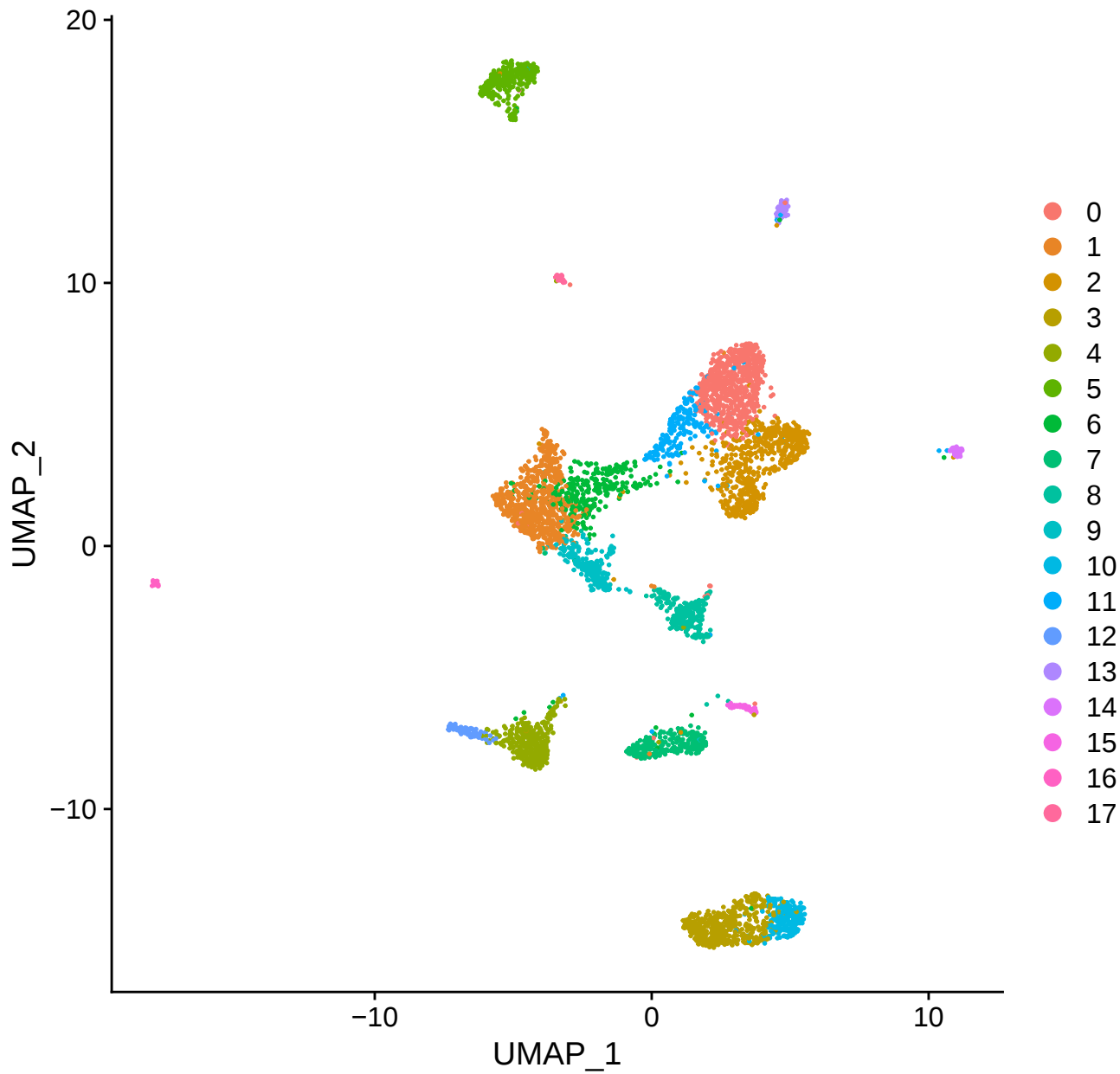
seurat_clusters
